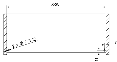
задня стінка шухляди
