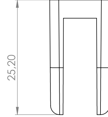
KESİT B-B
